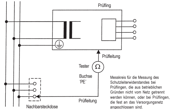
Messprinzipschaltung Schutzleiterwiderstand SK I, Bild C2
